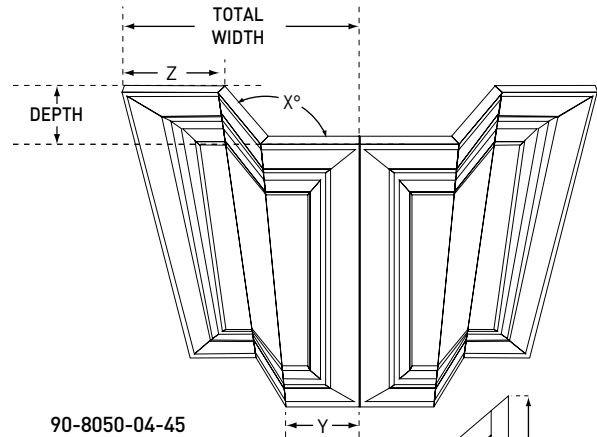
90-8050-04-45 «Z» doors
